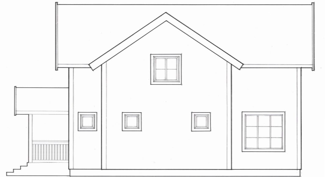
Västerfasad
